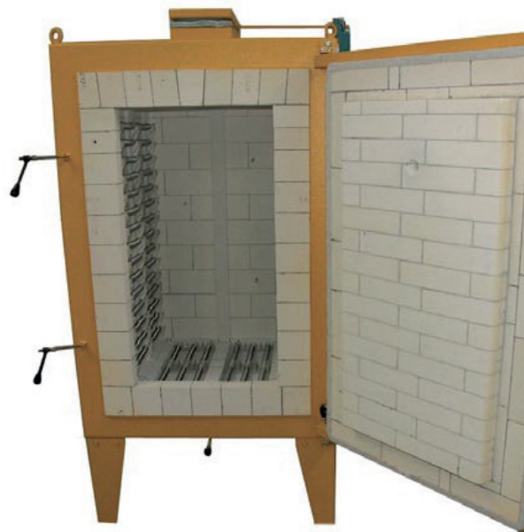
Four série H 300 litres spécial sculpture 1 m de haut sur demande
