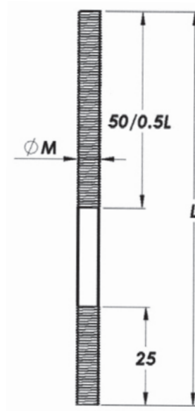
Tiges inox AISI-310 DRT
